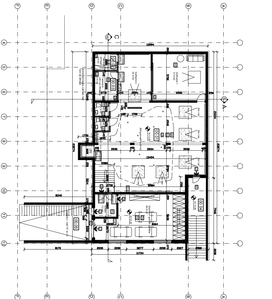
Grunnmynd kjallari - 1:100
